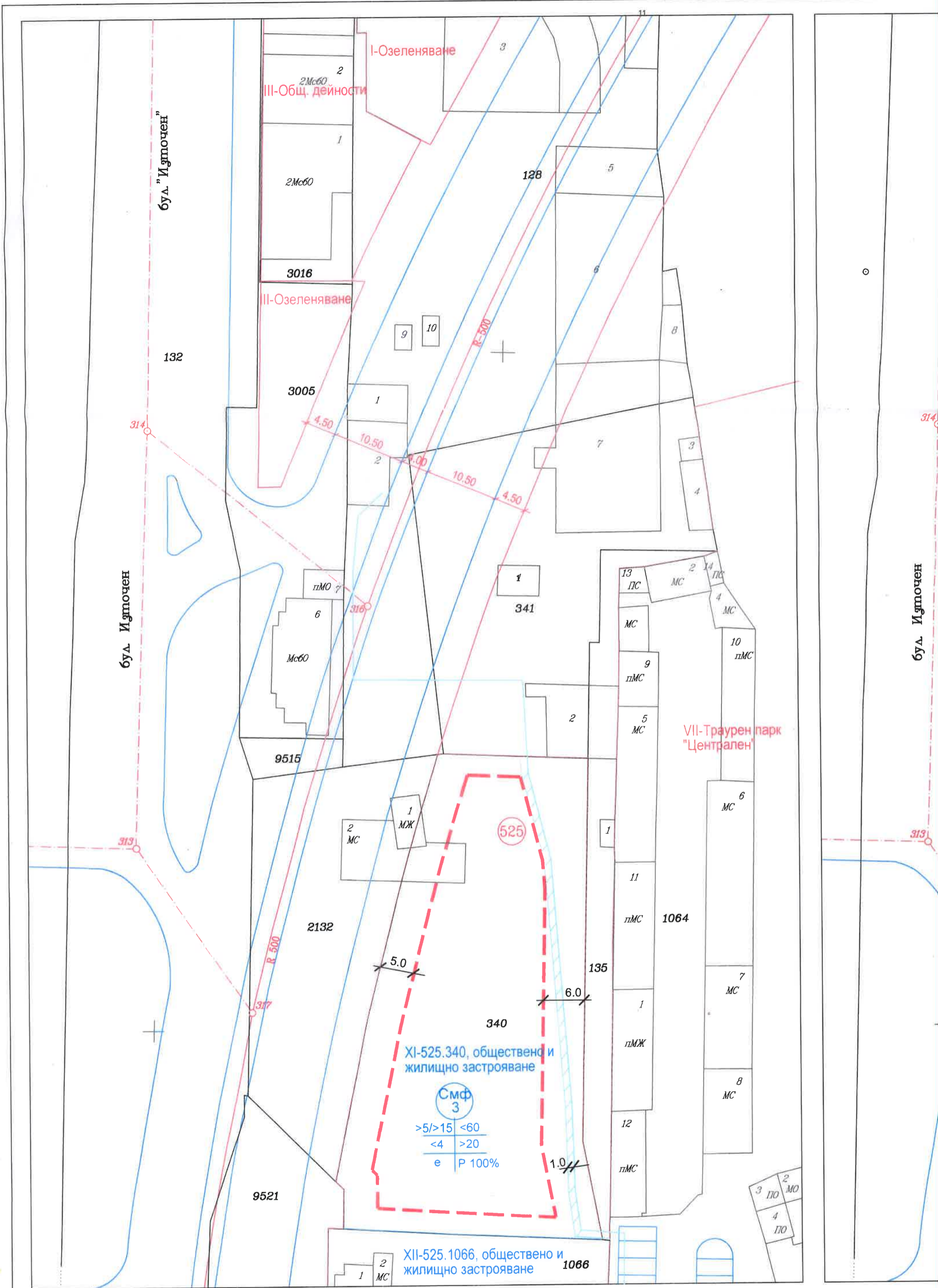
ИЗВЛЕЧЕНИЕ М 1:500 НА ЧАСТ ОТ КВ.525 ПО ПЛАНА НА ПЪРВА ГРАДСКА ЧАСТ-ЮГ ГР. ПЛОВДИВ ОДОБРЕН СЪС ЗАПОВЕДИ ИЗМЕНЕНИЕ № №№ОА-1022/ 01.06.1994Г., ОА-1456/ 18.06.2007Г. И 17ОА 2657/ 23.10.2017Г. НА ОБЩИНА ПЛОВДИВ И КАДАСТРАЛНА КАРТА, ОДОБРЕНА СЪС ЗАПОВЕД № РД - 18-48/ 03.06.2009Г. НА АГКК - СОФИЯ
